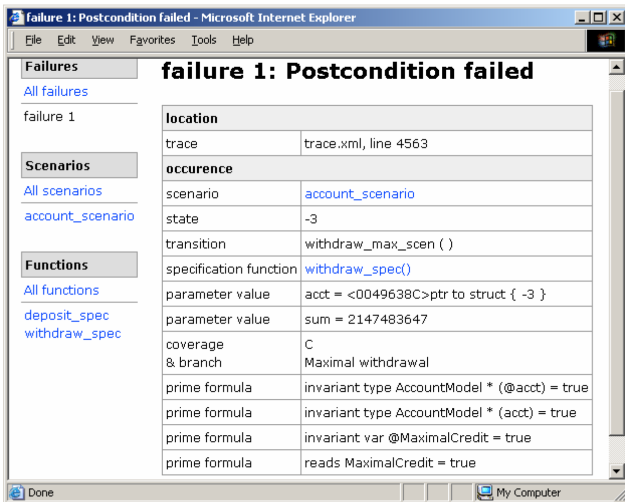
Рисунок 10. Подробный отчет об обнаруженном нарушении.
